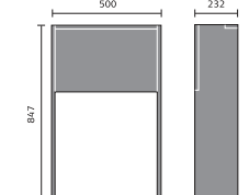
WC 500mm
