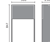
WC 500mm
