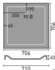
700mm Square
